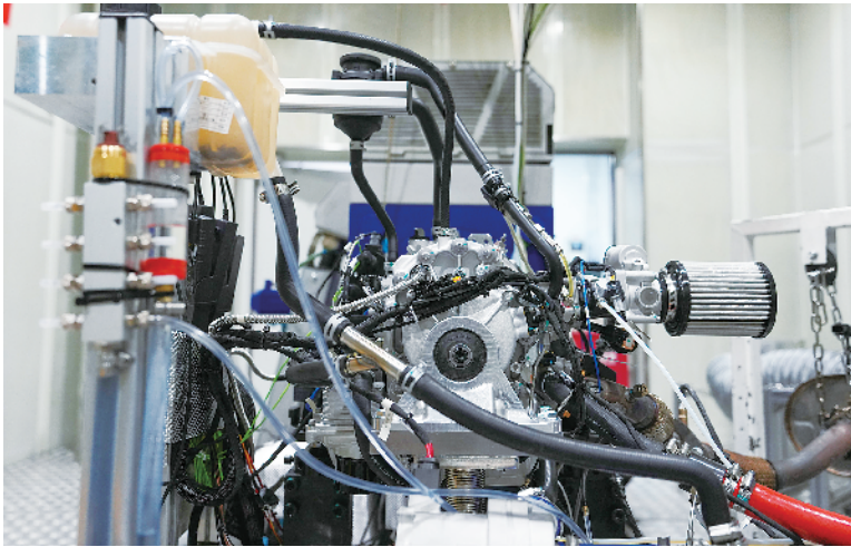
12 月 19 日拍摄的点火后的转子发动机 R05E 样机。
