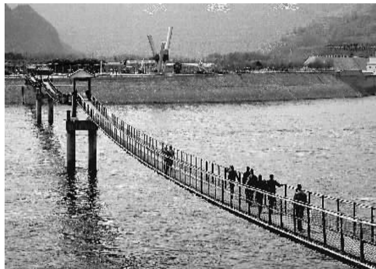
4月7日,游客在黄河小浪底水库参观。当日,黄河上最大的水利工程、“八五”期间国家重点建设项目——小浪底水利枢纽工程顺利通过国家竣工验收。作为黄河治理开发的关键性控制工程,小浪底工程控制了黄河92.3%的流域面积,90%的水量和近100%的泥沙,总库容126.5亿立方米。 新华社发
