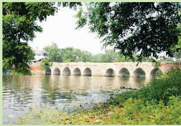
沈丘老城九拱桥，位于沈丘城关镇南关街泉河上。始建于清光绪十一年（1885 年），宣统三年（1911 年）重修，历百余年至今仍在使用。桥身南北向，长 56.2 米，宽 5.4 米，九拱，中拱略高，桥身
