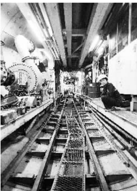
“万里长江地铁第一隧”将于9月底全部贯通 一名施工人员在地铁隧道施工间隙休息(8月21日摄)。截至8月23日,“万里长江地铁第一隧”左线盾构机掘进1756环,距终点仅剩472.5米,计划于9月30日到达汉口江汉路站,实现双线全部贯通。 由中铁隧道集团施工的这条越江地铁隧道位于武汉长江大桥和武汉长江公路隧道之间,是连接武昌、汉口两镇中心区域地铁2号线的过江通道,隧道全长约3100米,最大埋深48米。 新华社发
