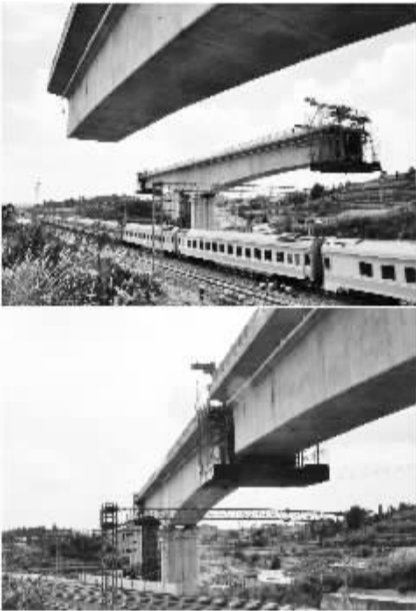
云南近万吨铁路桥梁“空中转体” 上、下图分别为沾益特大桥转体施工前与转体施工后(9月10日摄,拼版照片)。9月10日下午,经过1个小时的缓慢转动,矗立在沪昆铁路沾益火车站两侧、重达8300吨的两段“巨无霸”桥梁,向跨越的沾益火车站平转25.3°,实现桥梁精确合龙。沾益特大桥是沪昆高铁云南段的控制性工程。 新华社记者 潘洁 摄
